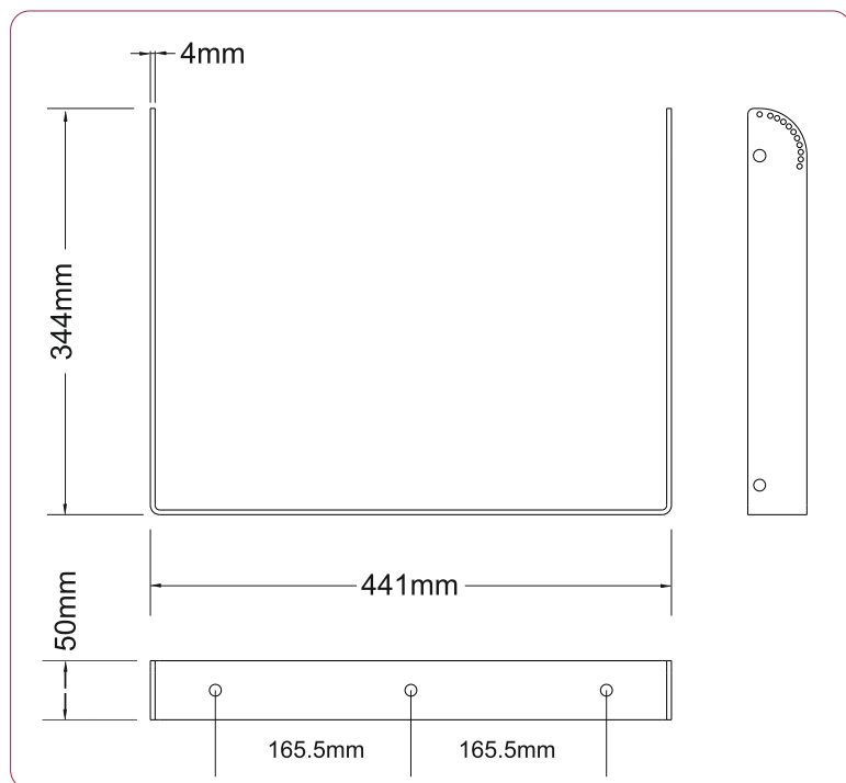
SUPPORT DE FIXATION MURALE POUR MODELES 112HC / EN - 112CT / EN - 112HCT / EN
