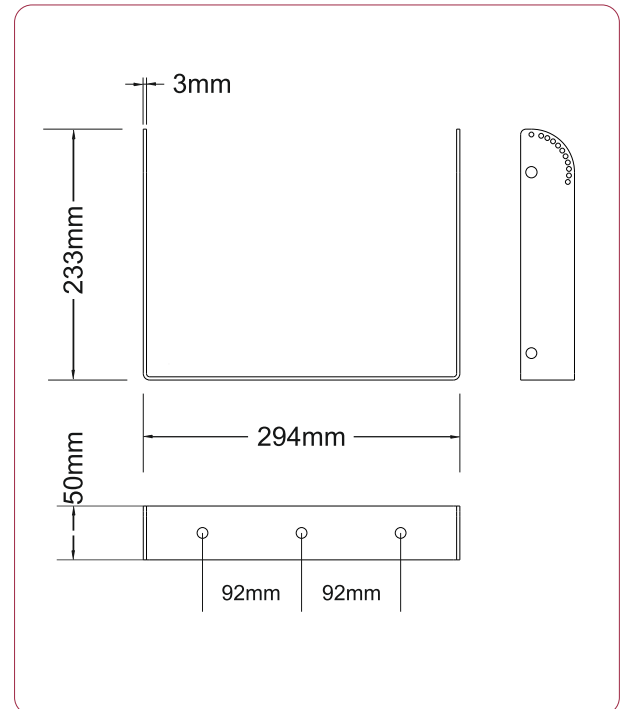
WANDBEFESTIGUNGSSTÜTZE FÜR MODELL 108CT / EN
